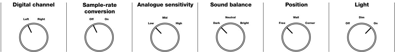
Пример настроек на задней части Confidence 20A
