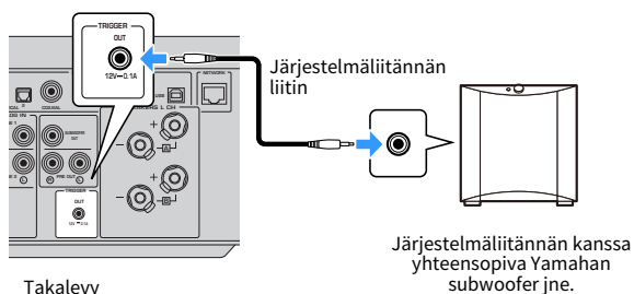
TRIGGER OUT-liittimet
